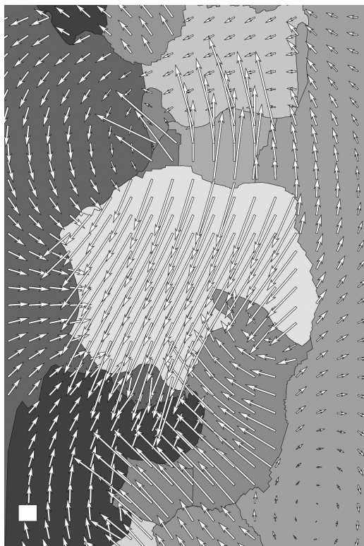
Les vitesses des 12 grandes plaques tectoniques (carte en projection cylindrique) Crédits: Christophe Vigny, chercheur CNRS
